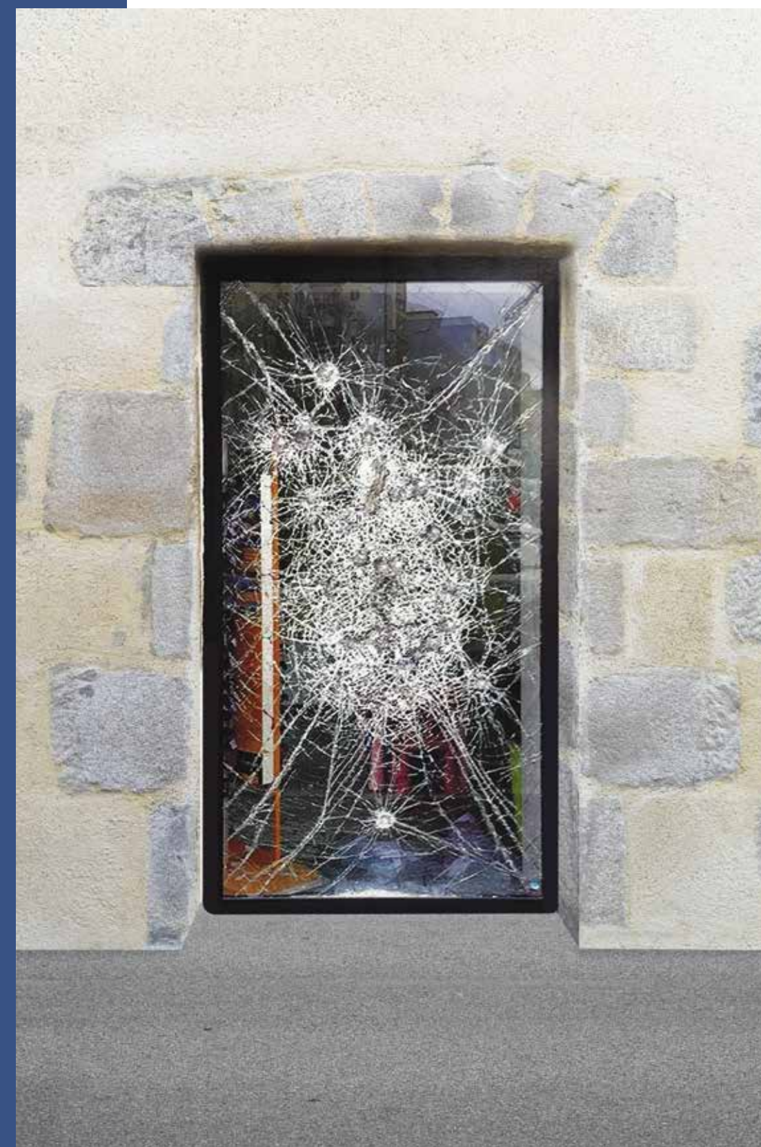
Résistance du vitrage face à des coups de marteau répétés
